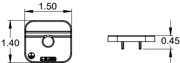
2) TOP PLATE
