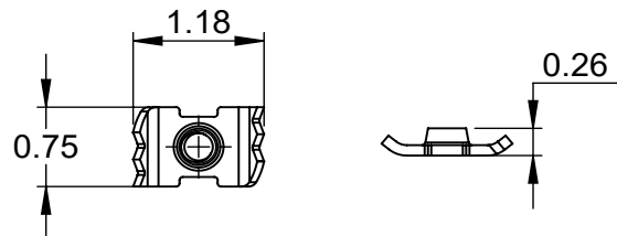
4) T-NUT, SHEET METAL
